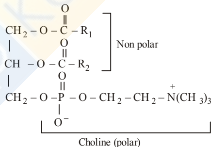
Fig. : Lecithin.
